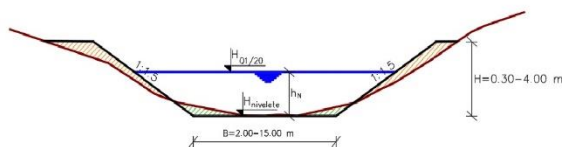
Карактеристични попречни профил канала
