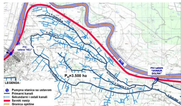
Прегледна карта Подсистема унутрашње одводње уз ПС Долина
